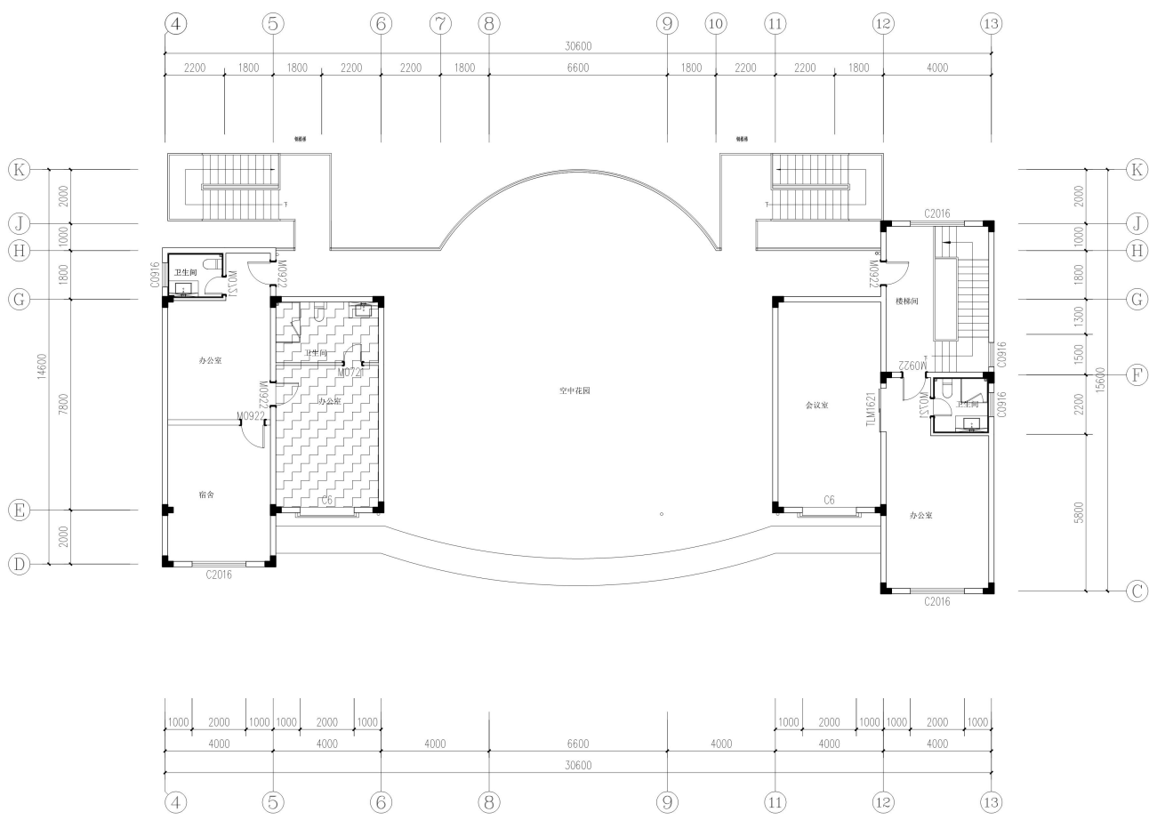
1 三层平面布置图 — LAYOUT PLAN 1:100
