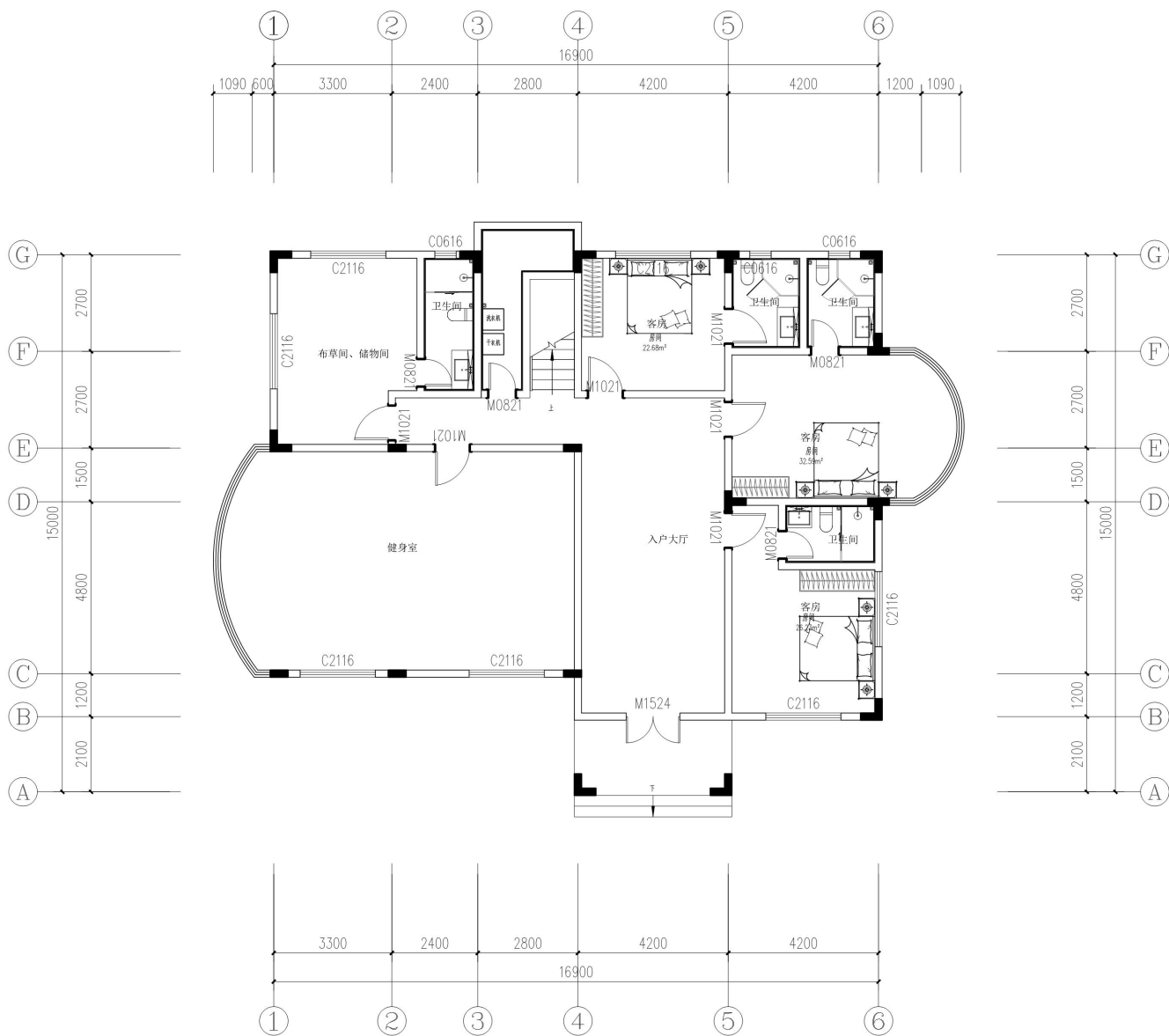
1 一层平面布置图 — LAYOUT PLAN 1:100
