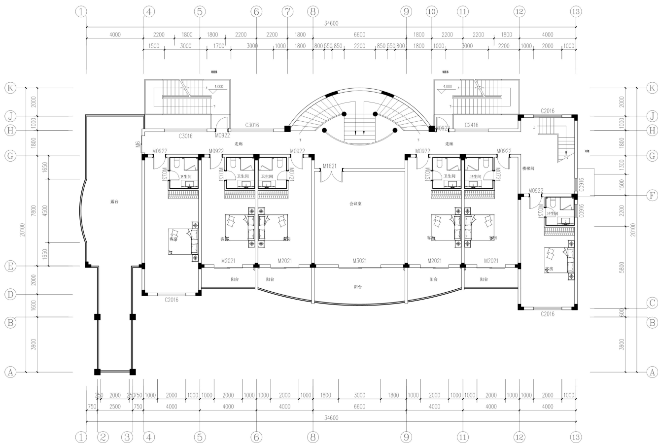
1 二层平面布置图 — LAYOUT PLAN 1:100
