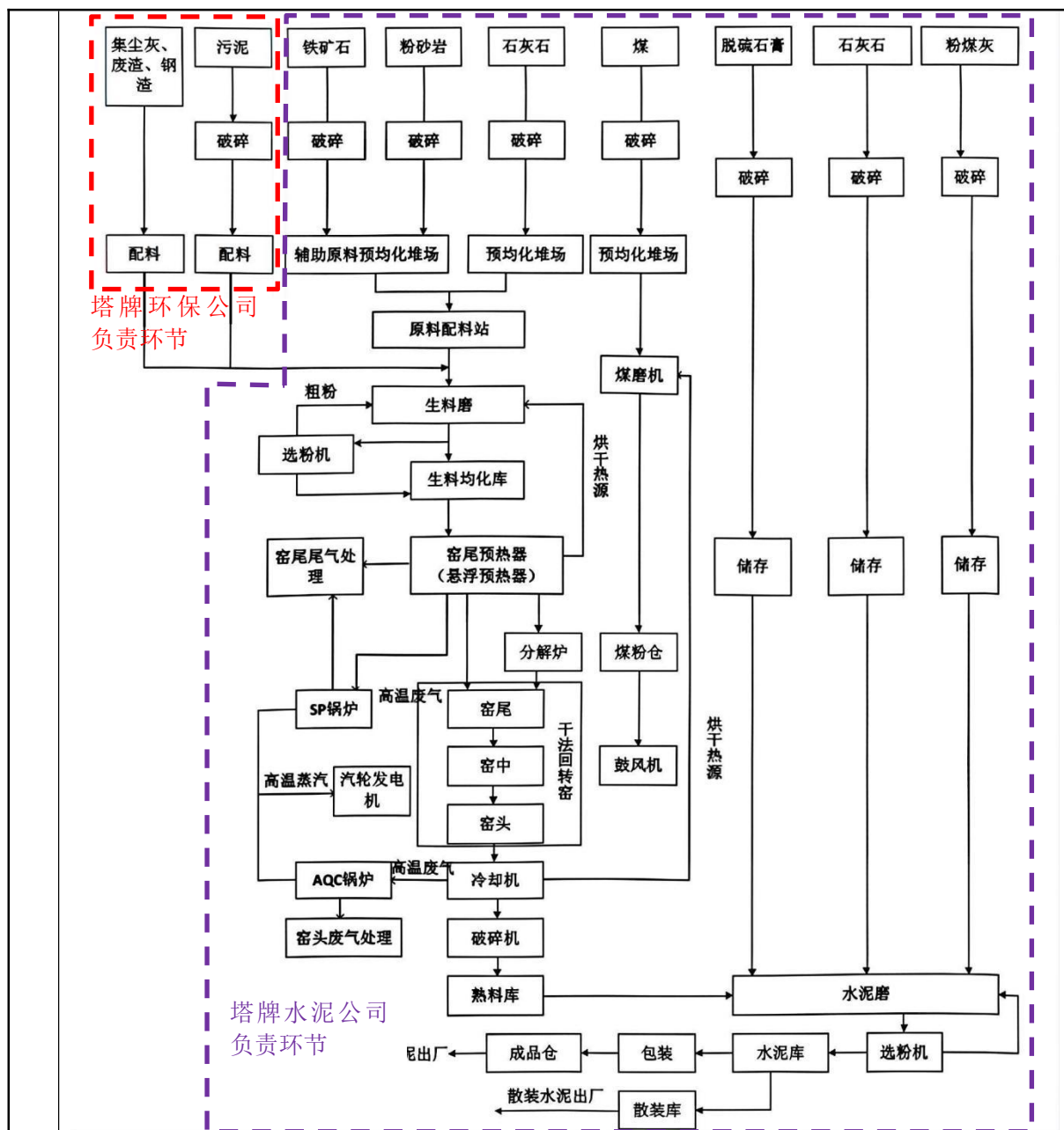
图 3 塔牌水泥厂区总工艺流程图
