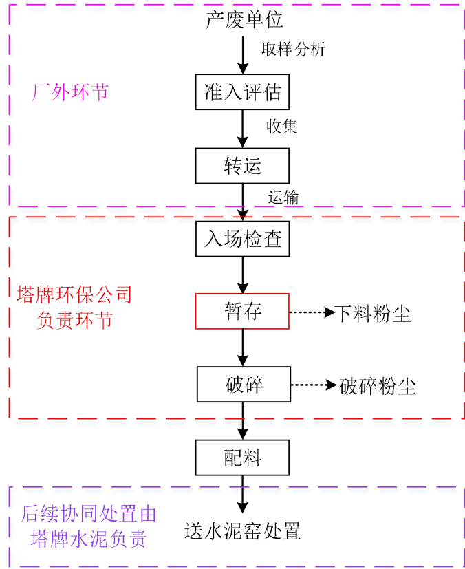
图 2 塔牌环保公司协同处置流程及产污节点图
