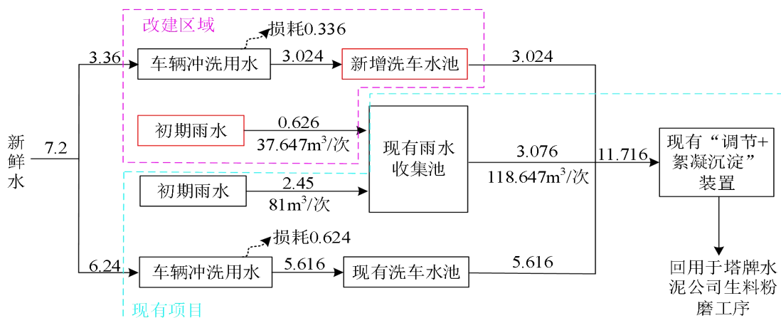
图1 项目建成后水平衡图 (单位: t/d)
